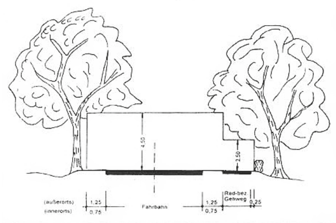
Lichtraumprofil
